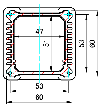
A-A ( 1 : 2 )
