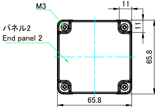
A-A ( 1 : 2 )
